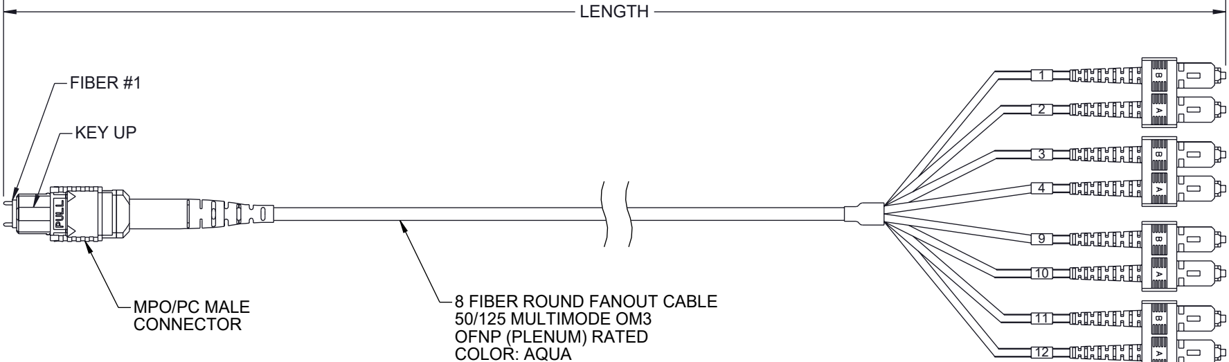
WIRING MAP TYPE A
